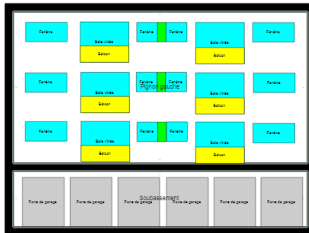
Pignons gauche du bâtiment n 4
